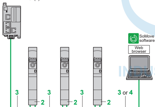
ATV320 Book + VW3A3616 module
