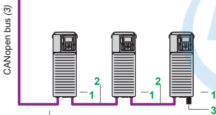
Altivar Process + VW3A3608 module
