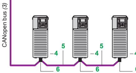
Altivar Process + VW3A3618 module
