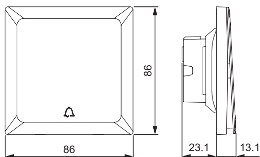
Bell Press Switch
