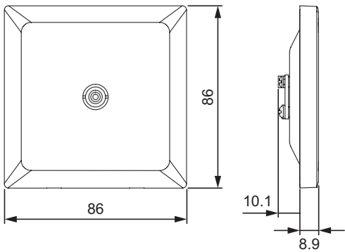
1G TV Socket – 75 Ohm
