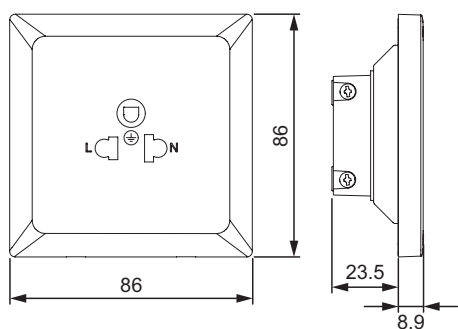
1G Universal Socket
