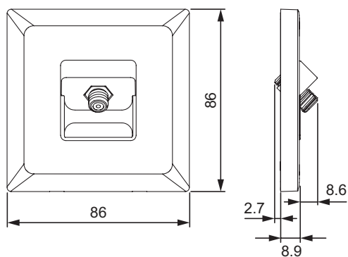
1G Cable TVF Connector
